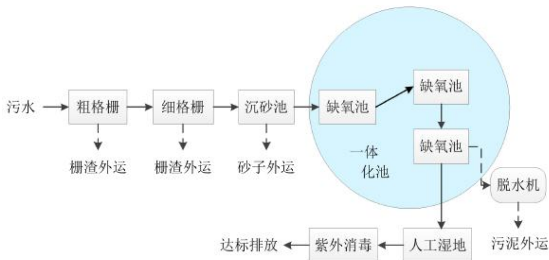
图 4-2 连山县城污水处理厂工艺流程
