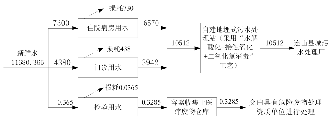
图 2-1 扩建项目给排水平衡图（单位：t/a）
