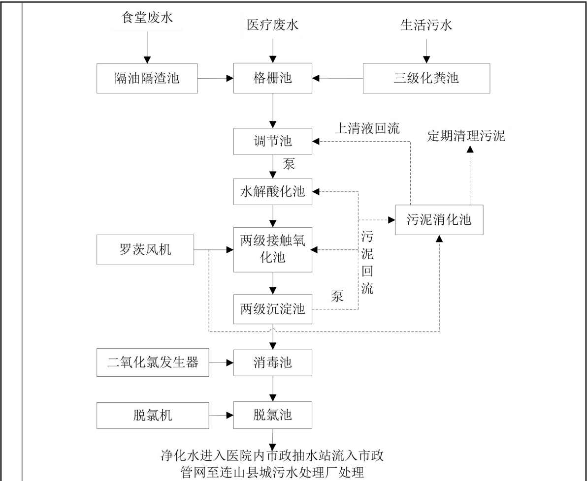
图4-1 项目自建地埋式污水处理站处理工艺流程
