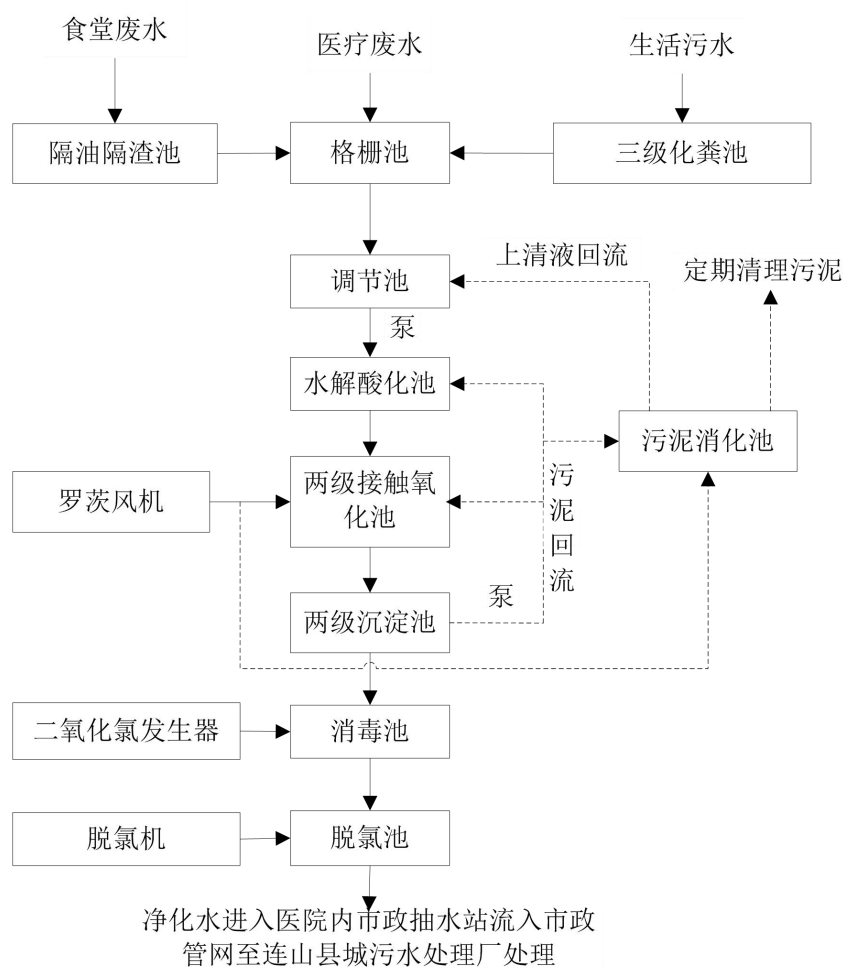
图 2-6 原有项目混合污水处理工艺流程图
