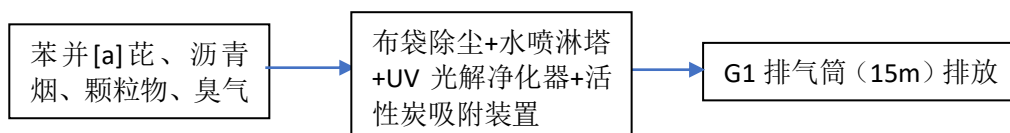
图4 沥青烟气、粉料搅拌粉尘处理工艺流程图
