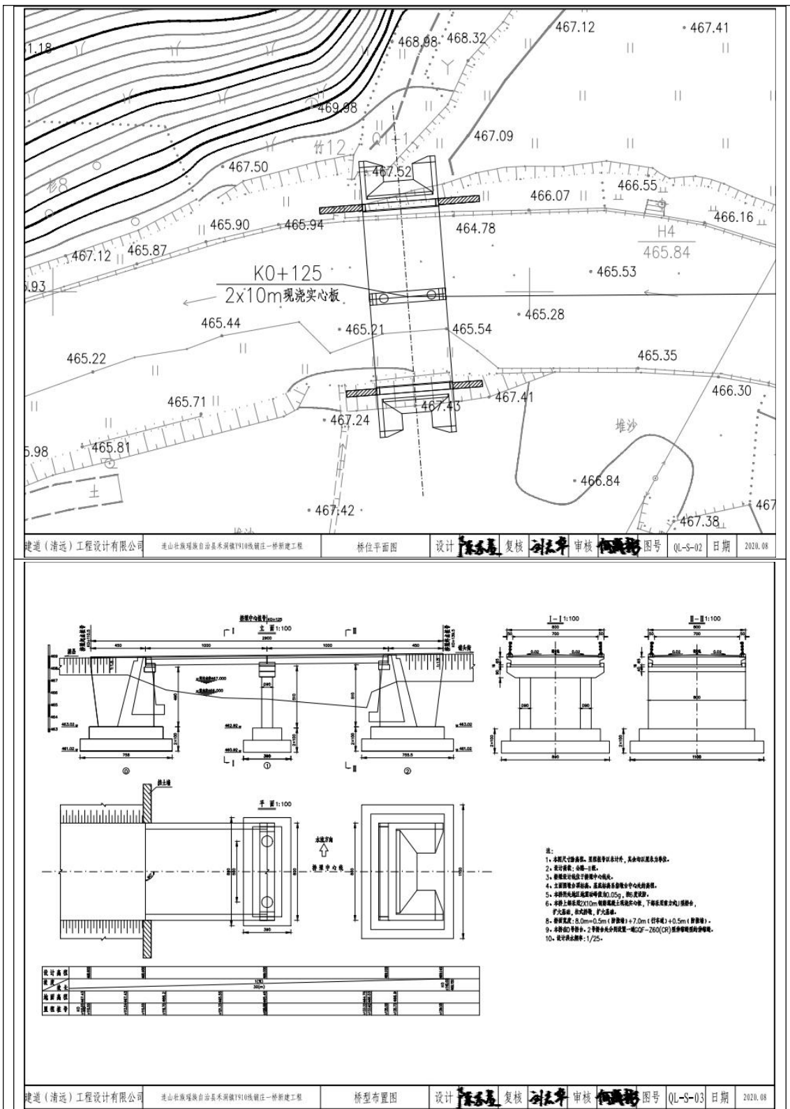
图1-1 桥梁整体设计
