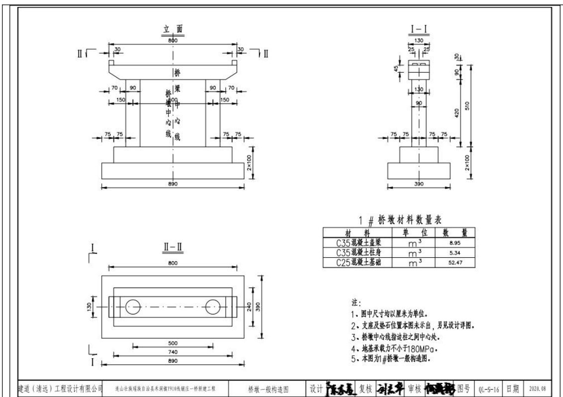
图1-3 桥台、桥墩构造图
