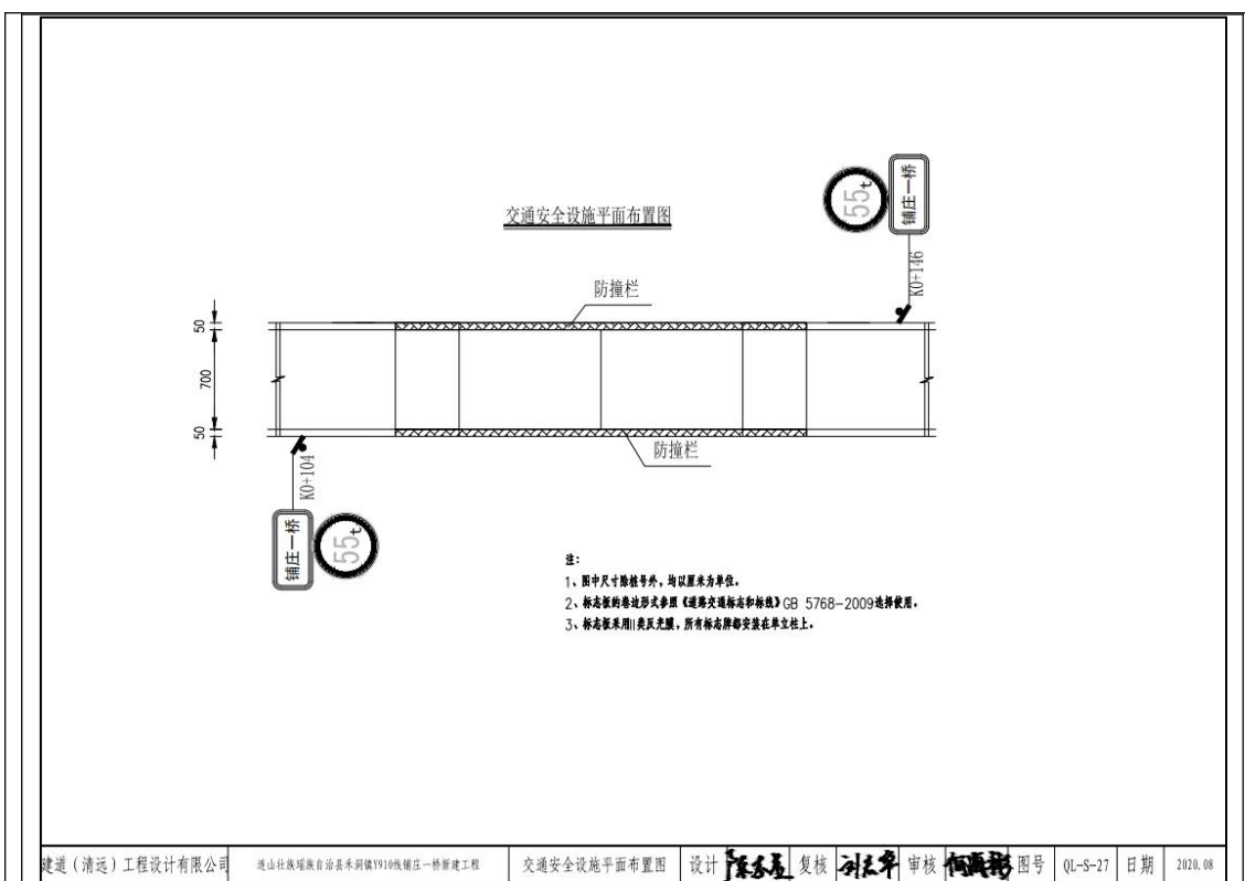
图1-4 交通安全设施平面布置图
